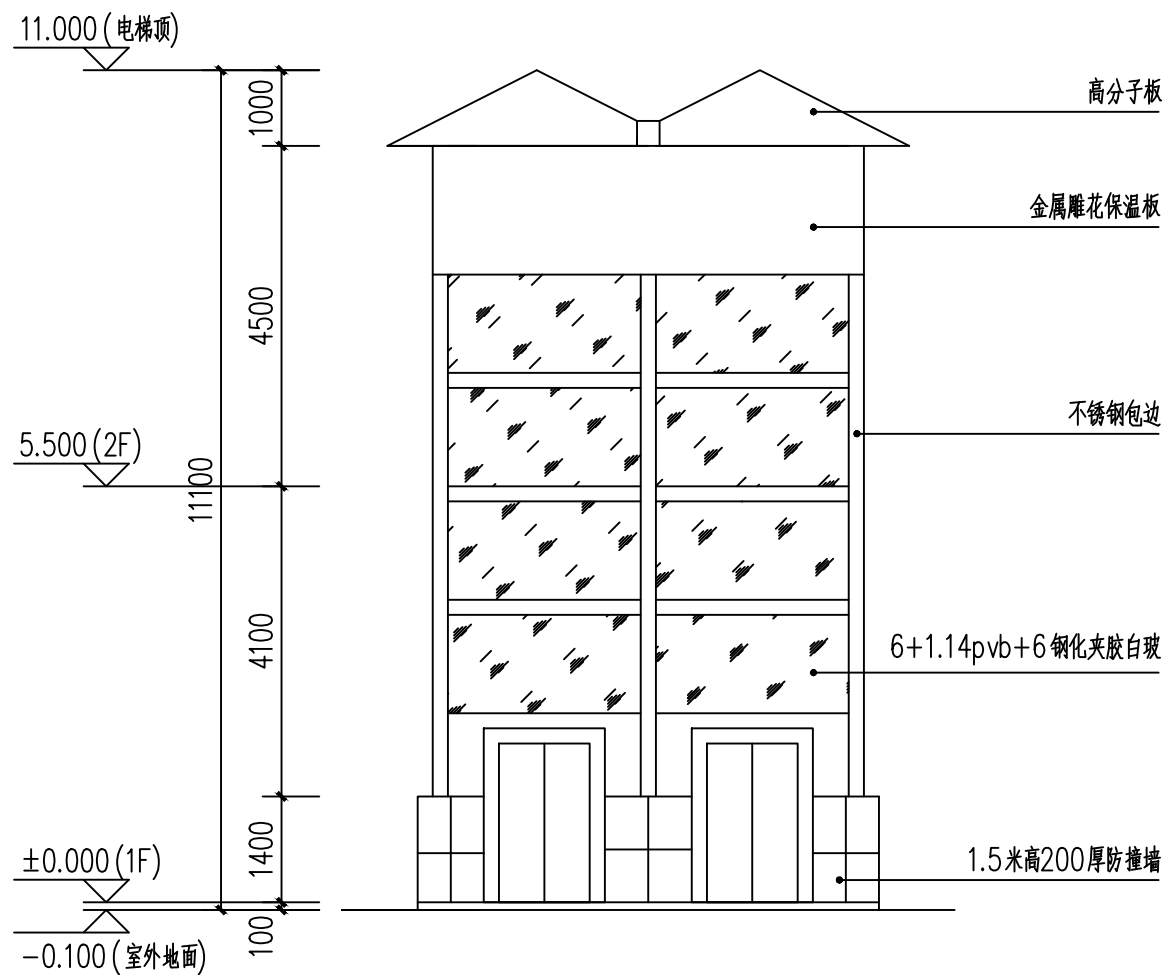
正立面 1:100
