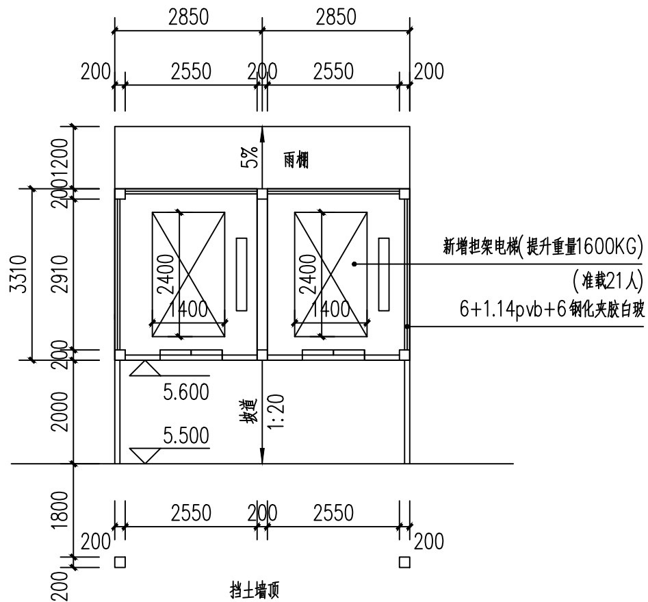
二层平面图 1:100
