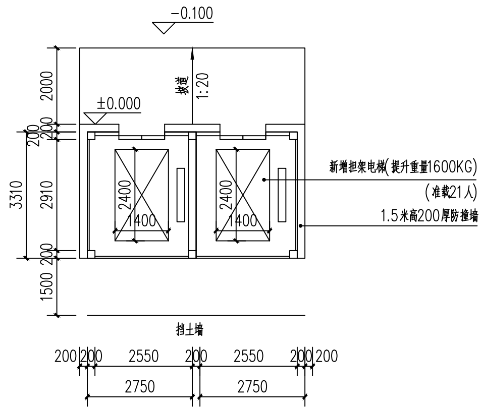
一层平面图 1:100
