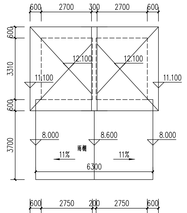
电梯顶平面图 1:100
